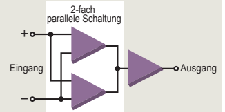
MCS+-Schaltungsarchitektur
